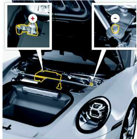
Fig. 22 : Bornes de la batterie au lithium
