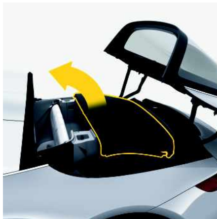
Fig. 228 : Fermeture de l'élément de capote
