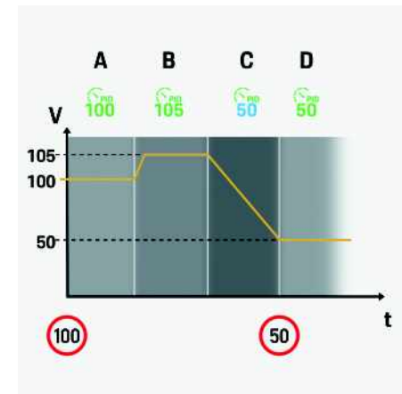
Fig. 171 : Exemple « Prendre en compte limites de vitesse » activée
