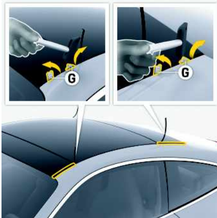
Fig. 237 : Extraction des supports rotatifs
