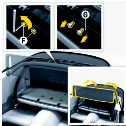
Fig. 46 : Escamotage du saute-vent
