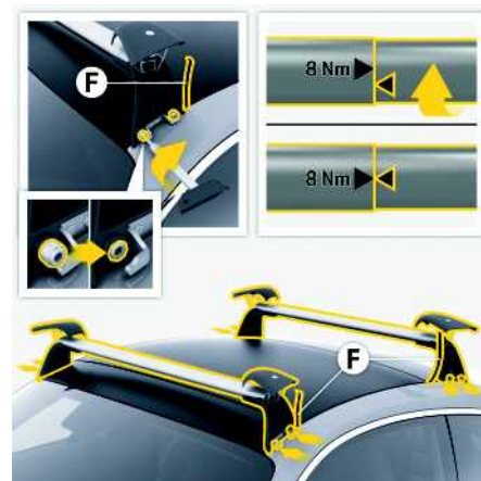
Fig. 242 : Serrage des vis sur le dessous du support
