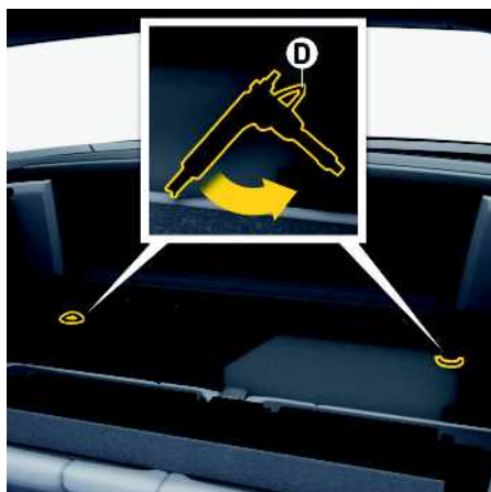
Fig. 224 : Déverrouillage de la lunette arrière en verre
