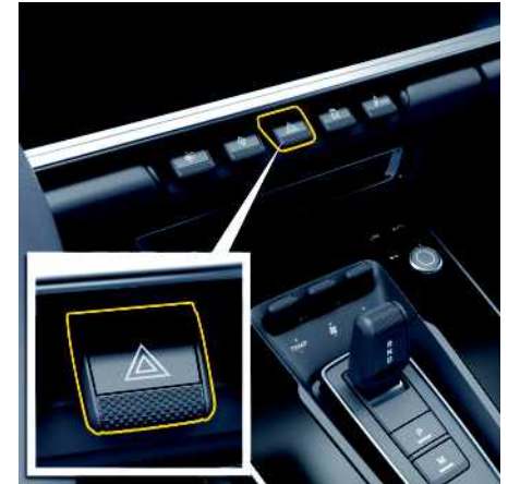
Fig. 100 : Allumage / Extinction des feux de détresse
