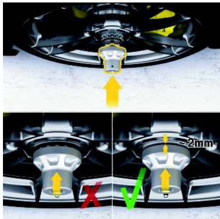
Fig. 134 : Mise en place de la douille
