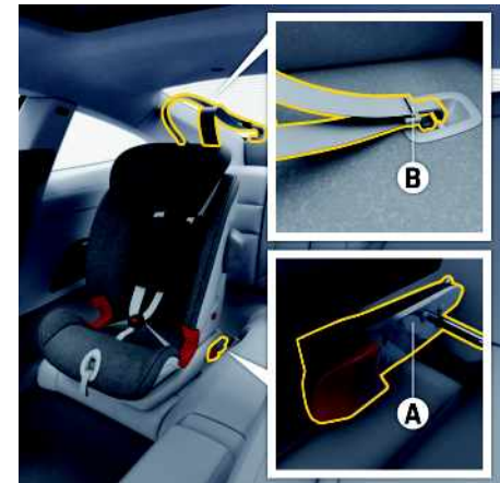
Fig. 256 : Installation d'un système de retenue pour enfants avec sangle d'ancrage (Top Tether)
