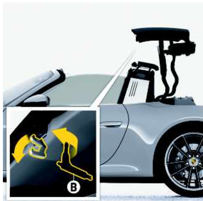
Fig. 230 : Déploiement du crochet de verrouillage
