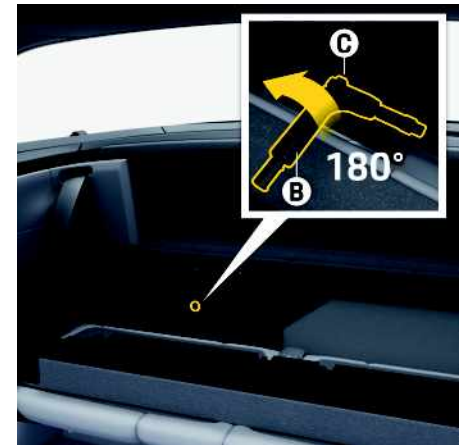
Fig. 223 : Dépressurisation du mécanisme du toit
