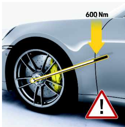
Fig. 144 : Serrage de la vis centrale
