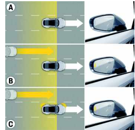
Fig. 10 : Un véhicule s'approche rapidement
