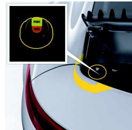
Fig. 116 : Indicateur du vase d'expansion
