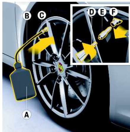
Fig. 89 : Injection du produit anticrevaision
