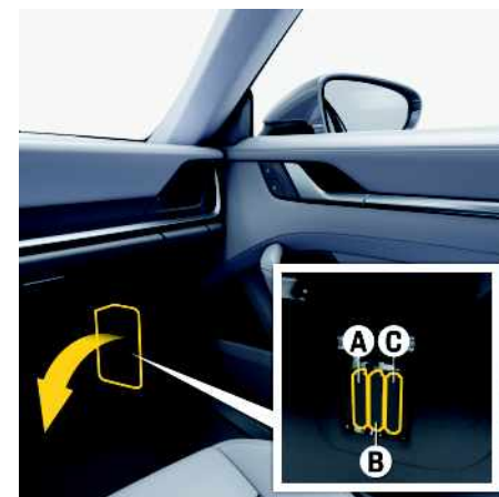
Fig. 108 : Boîte à fusibles côté passager
