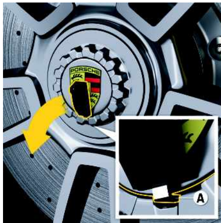
Fig. 132 : Extraction du bouchon obturateur à l'aide de l'outil auxiliaire
