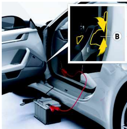
Fig. 37 : Déverrouillage d'urgence du capot du coffre à bagages - Raccordement de la borne moins
