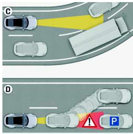
Fig. 167 : Entrées/sorties de virage (C) et véhicules à l'arrêt (D)
