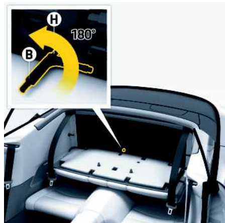
Fig. 47 : Dépressurisation du mécanisme de la capote
