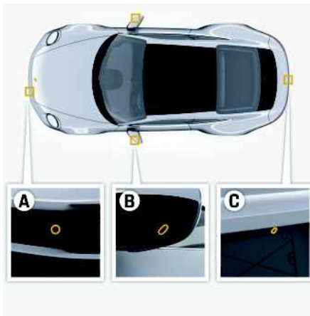
Fig. 18 : Emplacement des caméras périphériques
