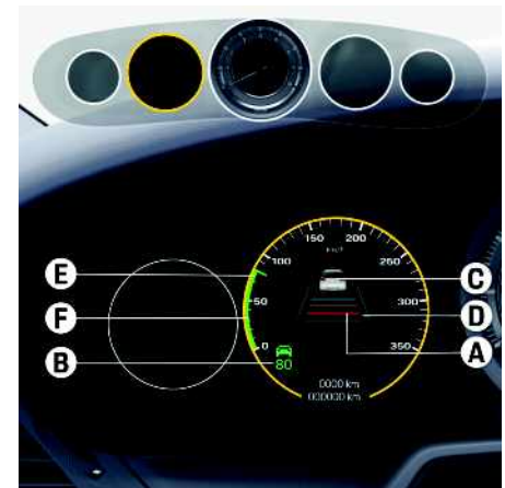
Fig. 198 : ACC dans l'affichage Vitesse et assistance
