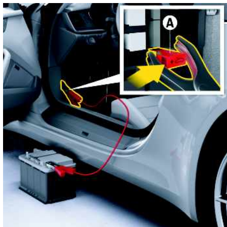
Fig. 36 : Déverrouillage d'urgence du capot du coffre à bagages – Raccordement de la borne plus
