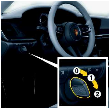
Fig. 92 : Positions de la clé dans le contacteur d'allumage
