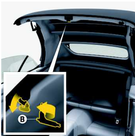
Fig. 57 : Déploiement du crochet de verrouillage
