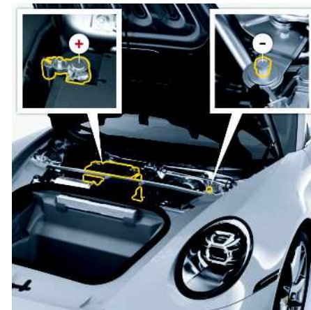
Fig. 6 : Bornes de la batterie au plomb
