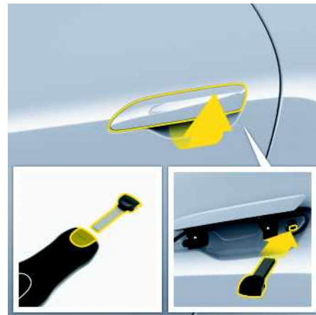
Fig. 270 : Déverrouillage / Verrouillage de secours
