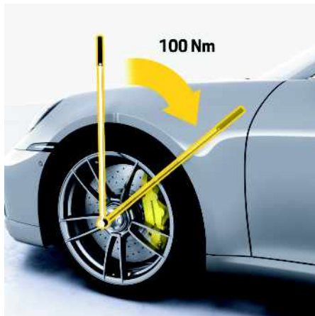
Fig. 149 : Serrage de la vis centrale
