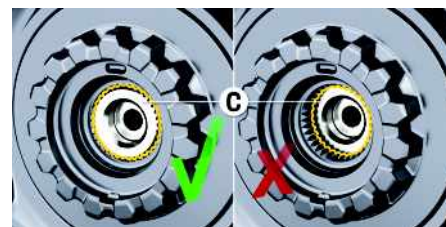
Fig. 146 : Contrôle du positionnement de l'axe de sécurité
