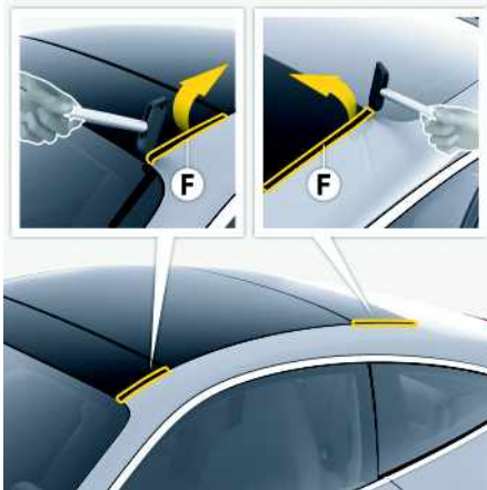
Fig. 236 : Retrait des joints de la rampe de pavillon
