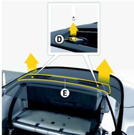
Fig. 45 : Retrait du capot des arceaux de sécurité
