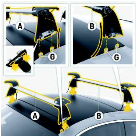
Fig. 240 : Adaptation de la longueur des supports
