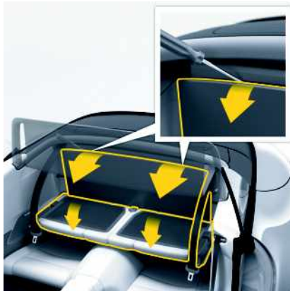
Fig. 41 : Rabattement des dossiers arrière et de l'habillage de tablier arrière vers l'avant
