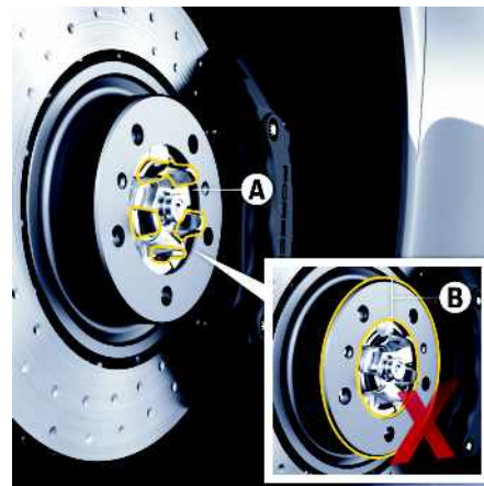
Fig. 126 : Surfaces de contact des roues
