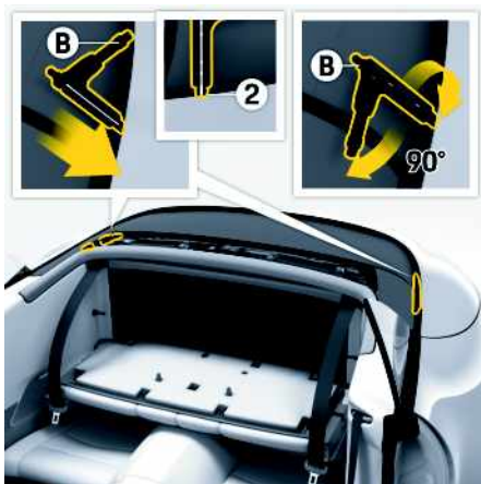
Fig. 50 : Déverrouillage du capot de puits de capote (étape 2)
