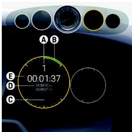
Fig. 66 : Chronomètre dans le combiné d'instruments
