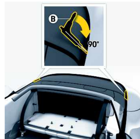
Fig. 49 : Déverrouillage du capot de puits de capote (étape 1)
