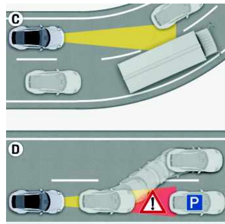
Fig. 195 : Entrées/sorties de virage (C) et véhicules à l'arrêt (D)
