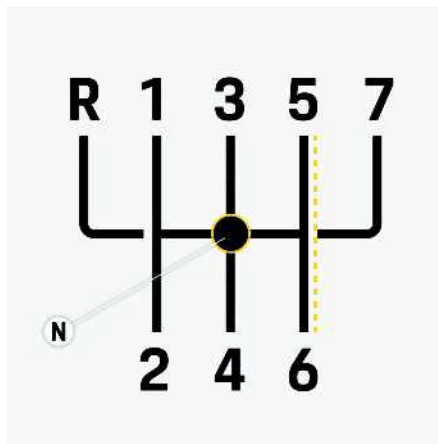
Fig. 27 : Position des rapports sur le levier de vitesses
