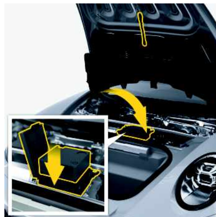
Fig. 83 : Mise en place du compresseur pour pneumatiques
