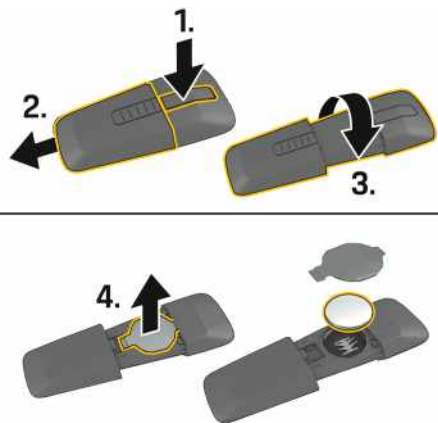
Fig. 175 : Remplacement de la pile de la carte conducteur PVTS Plus
