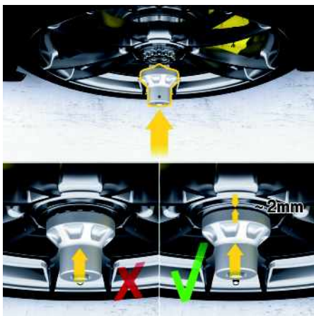
Fig. 143 : Mise en place de la douille
