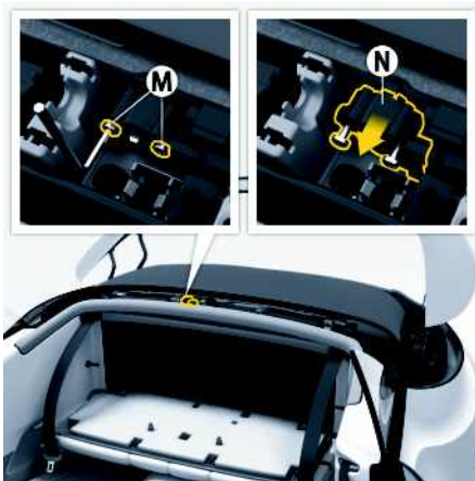
Fig. 53 : Desserrage des vis et retrait de l'unité de transmission du moteur vers l'avant
